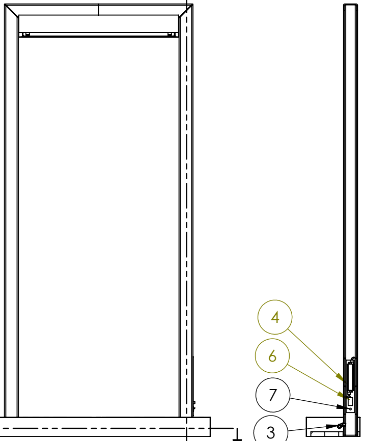
SECTION A-A SCALE 1 : 28
